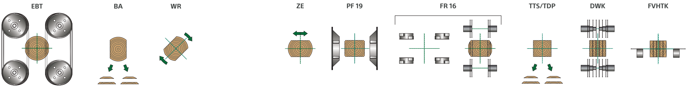
Einschnitt-Modus bei Schnittbildern mit 4 Seitenbretter im Nachschnitt
